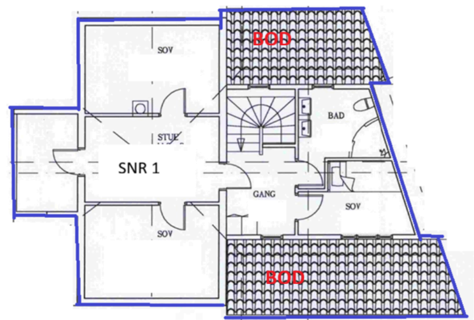
Seksjonseringstegning snr 1 Thomasløkken 4, 2.etasje gnr 324 bnr 129 Asker
