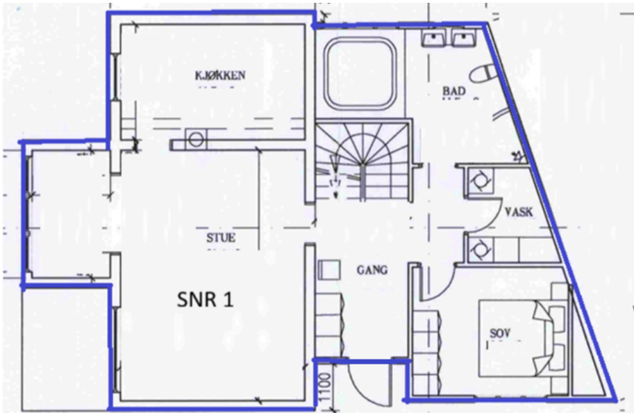
Seksjonseringstegning snr 1 Thomasløkken 4, 1.etasje gnr 324 bnr 129 Asker
