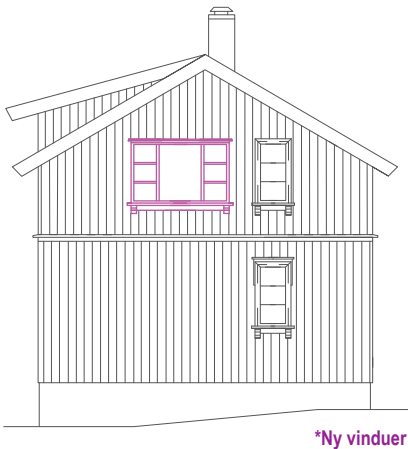
Ny fasade syd
