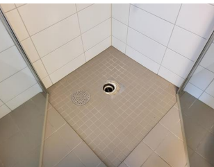
Tettesjiktets tilslutning til sluk - Sluk 2
