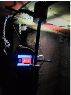
Stikktaking i treverk, fukt og fuktmålinger - Målinger i stubbloft og bjelker
