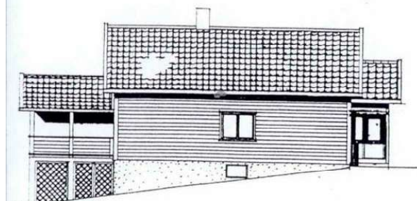
FASADE NORD
