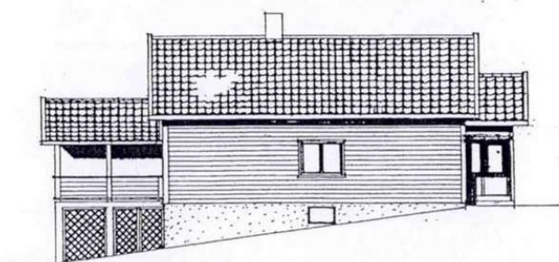
FASADE NORD
