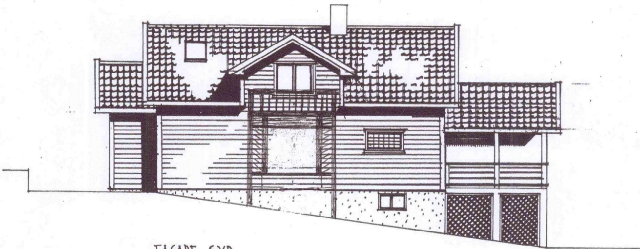
FASADE SYD
