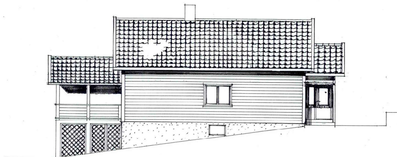
FASADE NORD
