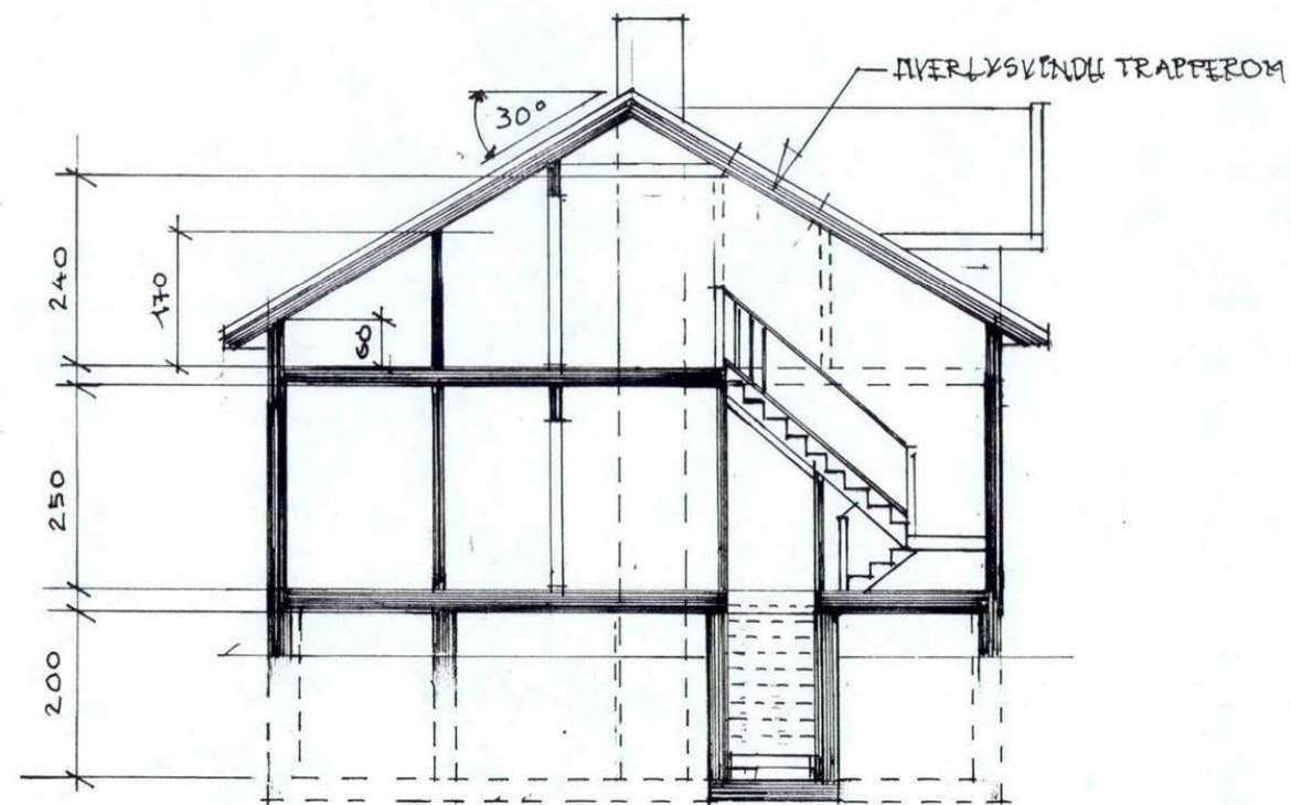
SNITT
