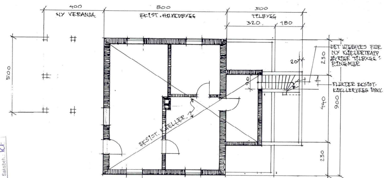
KJELLERPLAN
