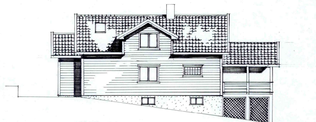
FASADE SYD
