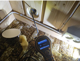
Kontroll i lukkede konstruksjoner - Fuktmåling i utlektet kjellervegg
